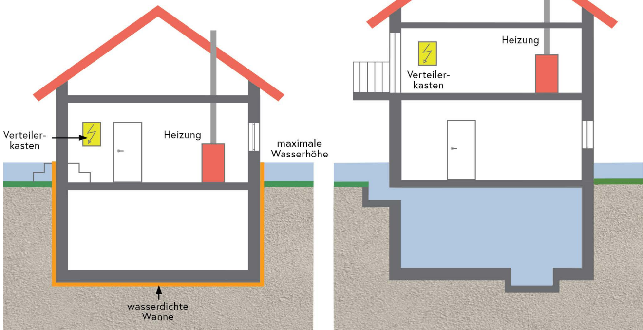
Abbildung 54: Hochwassersichere Installation von Stromverteiler und Heizanlage. Auf Ölheizungen sollte in hochwassergefährdeten Gebieten generell verzichtet werden.
