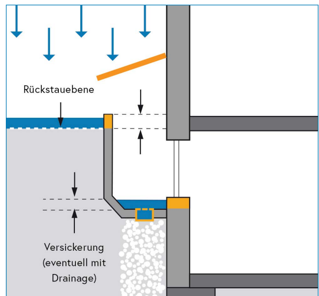
Abbildung 29: Richtig geschützter Lichtschacht (Schemaskizze). Befinden sich Dachrinnen oberhalb von Lichtschächten, sollten diese zusätzlich abgedeckt werden, damit kein Schwallwasser vom Dach in den Lichtschacht eindringen kann.
